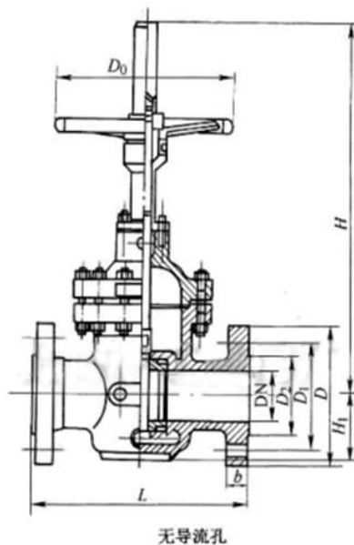
Type2- Z43WF/KZ43WF DN50~DN1000 2"~40" Class150
